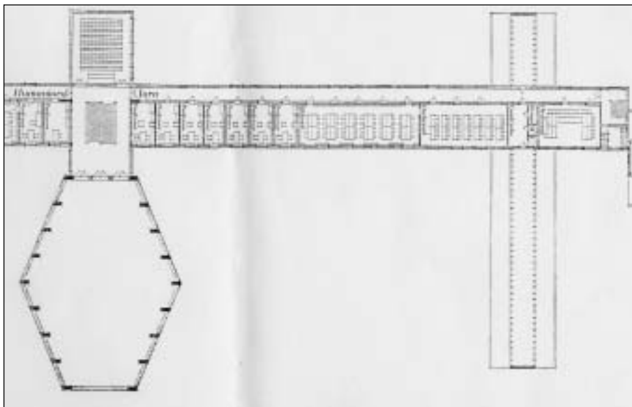
Plan over juragangen i den nye hovedbygning. Gengivet efter Arkitektens Maanedshæfte, XXXVI, 1949.
